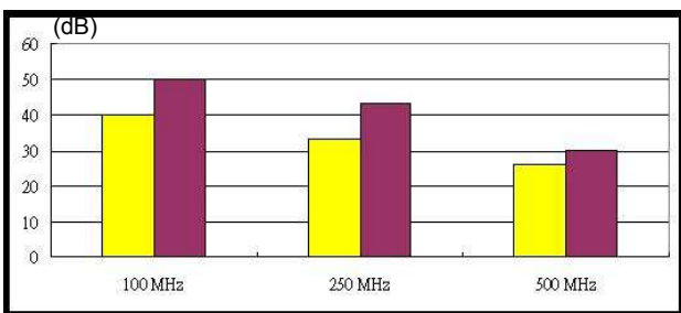
PSNEXT
